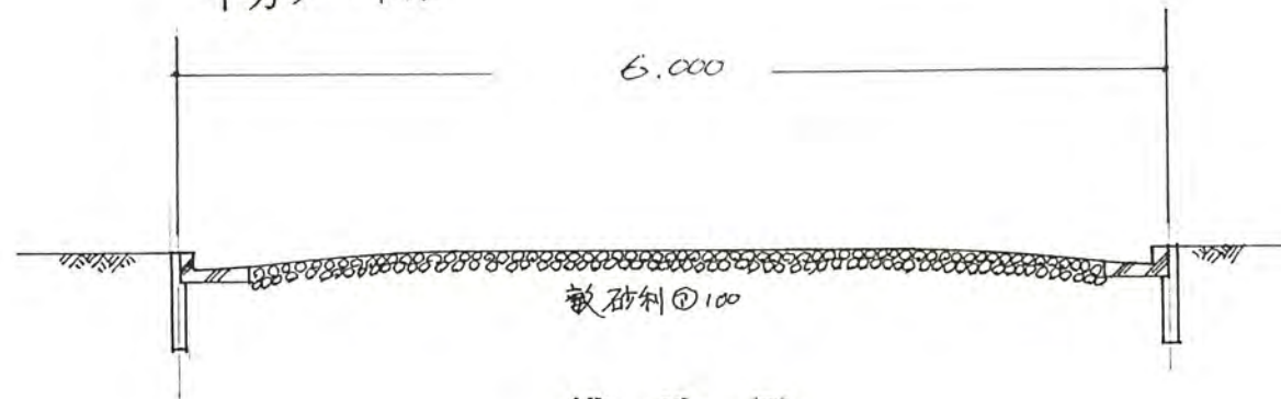
構造図
