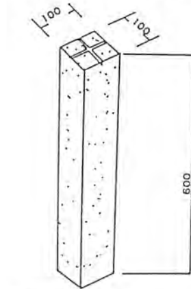
境界石 S=1/10
