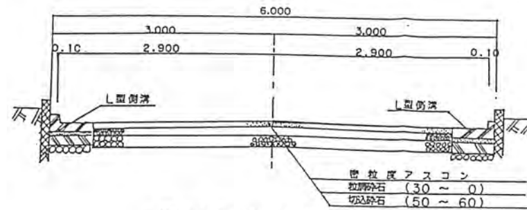
構造図 S=1/50
