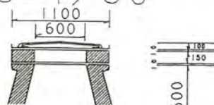
円形人孔構造図 S=1/50
