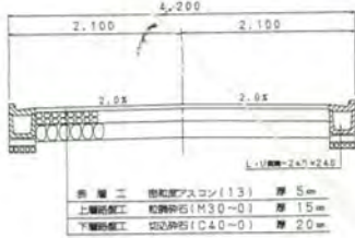
道路断面図 S=50
