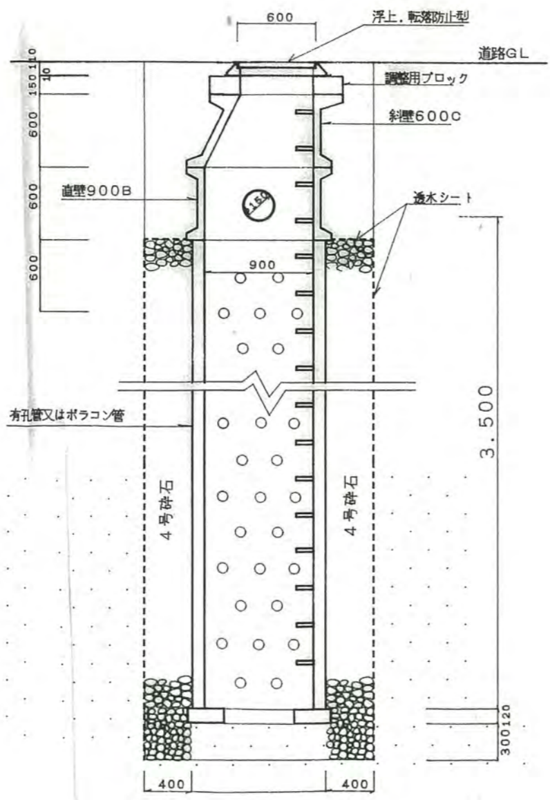
浸透井構造図
