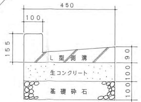
構造図 S=1/10
