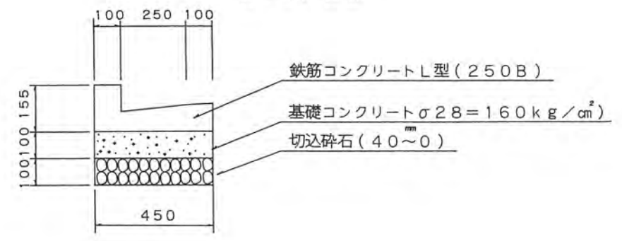
構造図
