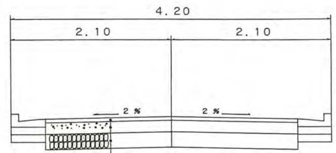
横断図
