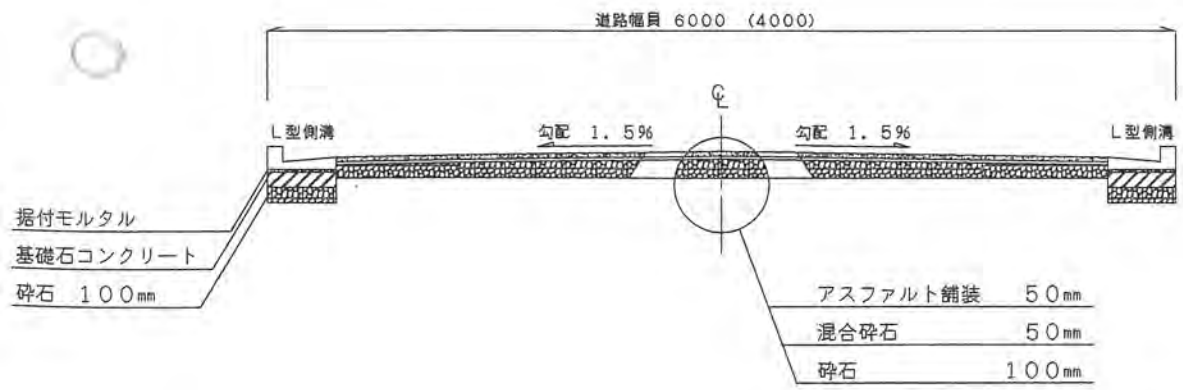
道路構造図 S = 1 : 50
