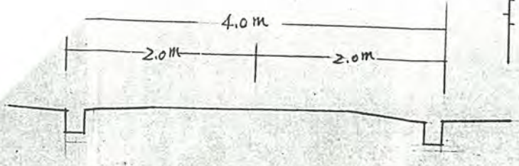
道路断面図
