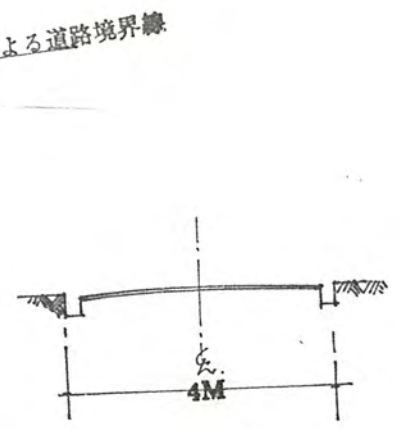
断面図 1 : 100
