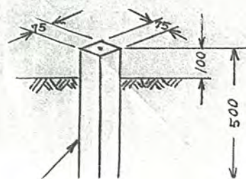
標石図
