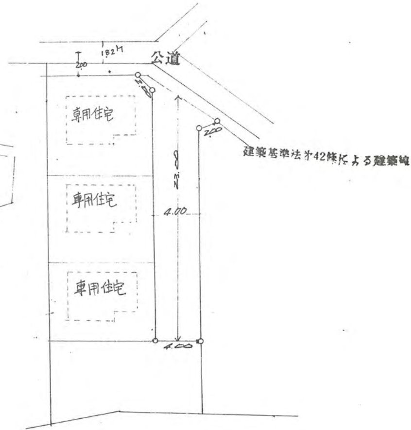
実測図 1/300
