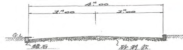
道路断面図
