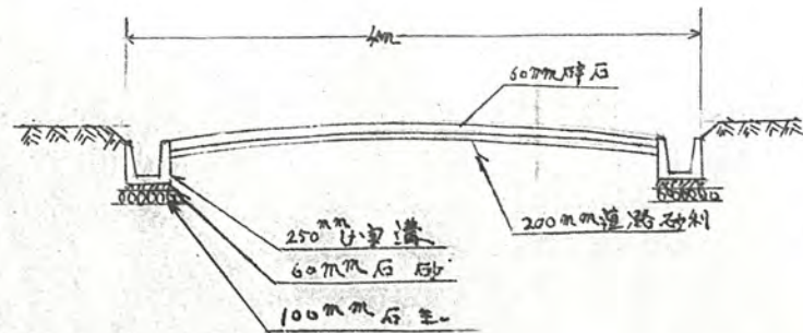
構造圖
