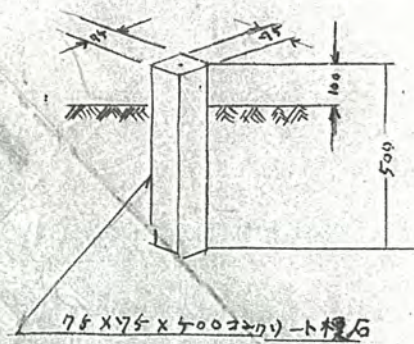
標石圖
