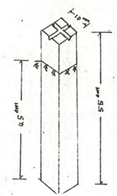
境界石 S=1/50
