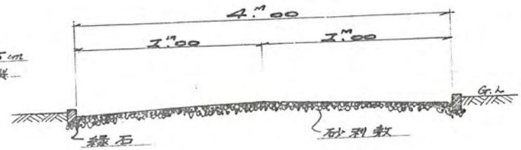
道路標識石柱断面図 Δ=1/50
