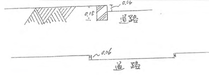
断面図
