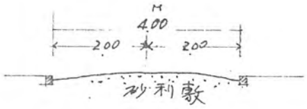
断面図
