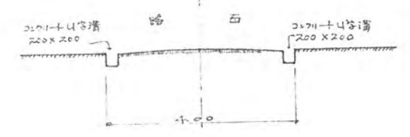
断面西図 S=100
