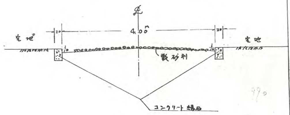
道路断面图 S 1/40
