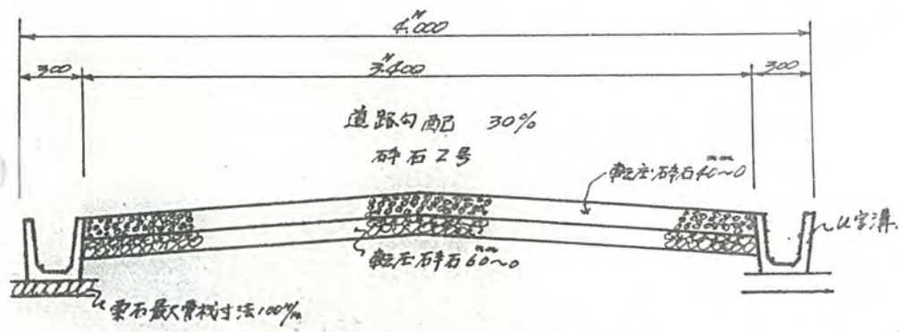
道路断面図繪尺 1=30
