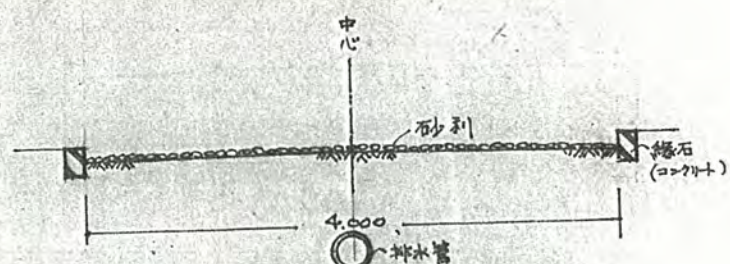
構造図 道路造成方法 1/50
