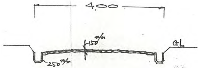
道路断面図
