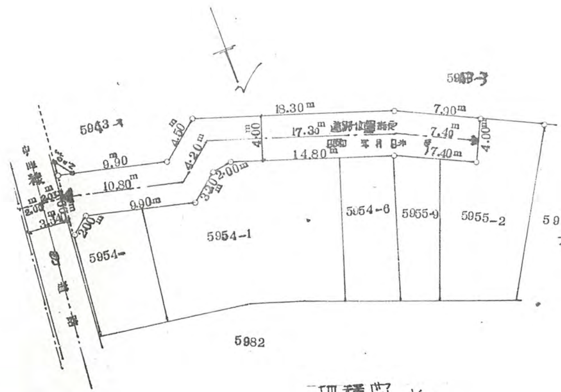
III 積込 1/300
