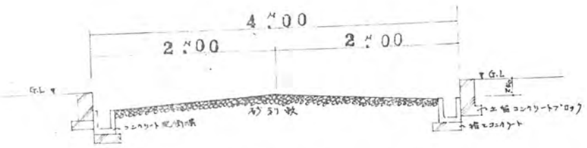
道路断面図 1/50
