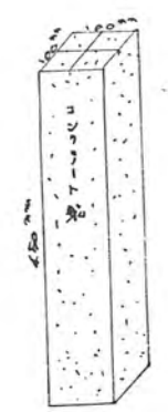
コンクリート 路標 鐵石柱 1/50
