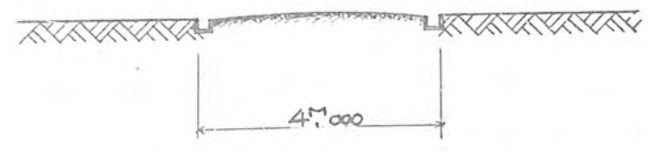
指定道路断面図
