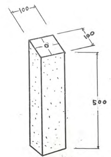
標杭・コンクリート製
