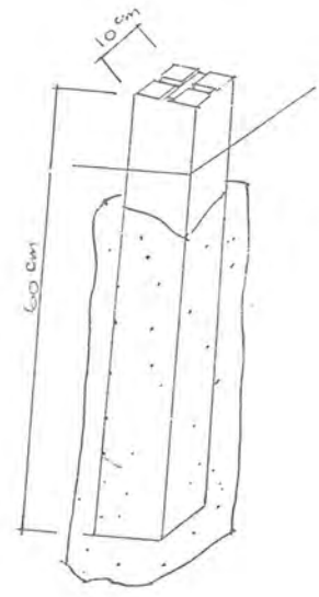
境界石構造図 S:1/10
