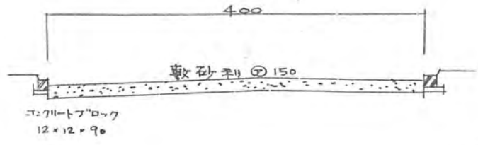
道路断面図 S:1/50
