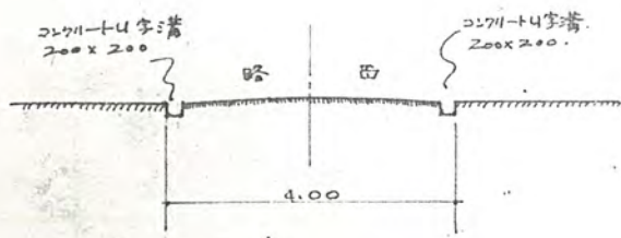
断面図 S=1/100
