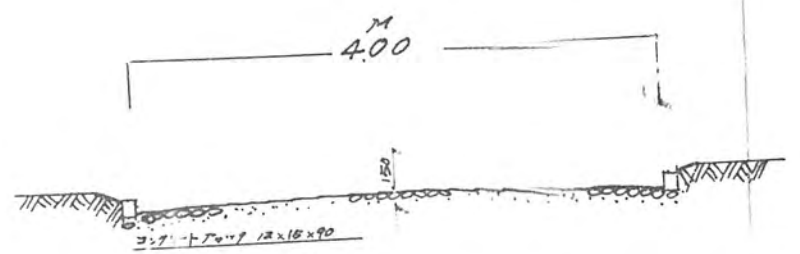
道路断面圖 S=1/50
