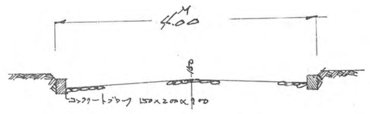
断面図
