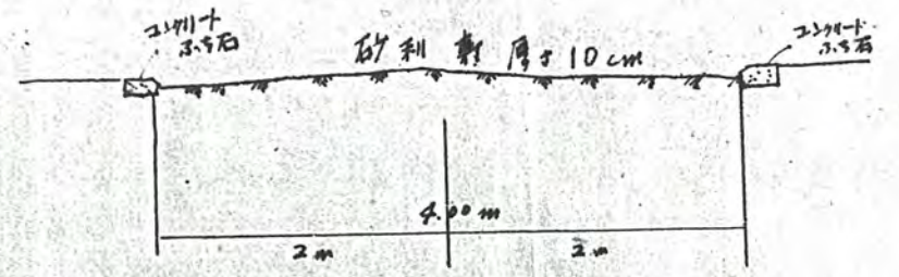
道路横断面図
