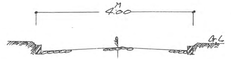
道路断面図
