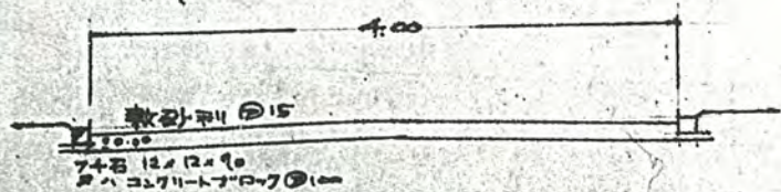
道路断面図 1/50
