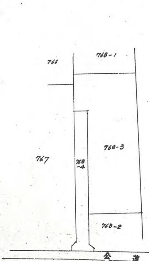
公図写 1/600
