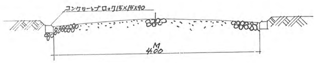
道路断面図 S=1:40
