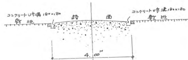
断面図 S1=100
