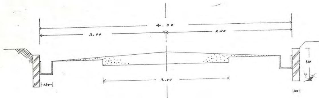
断面図 S \frac{1}{30}
