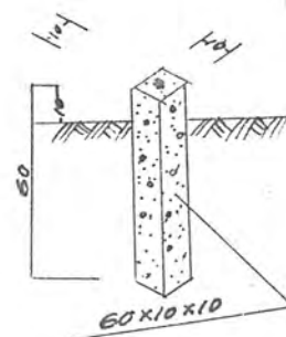
標杭図
