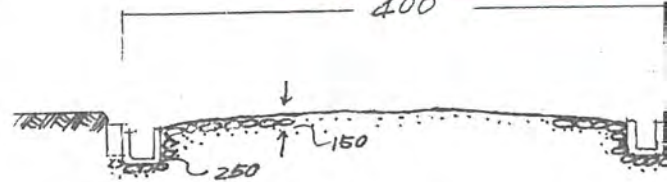
道路断面図
