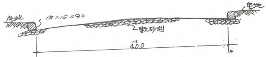
道路断面図 S 1/40
