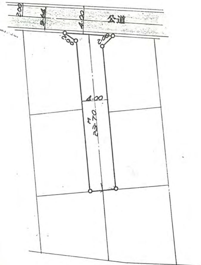
配置図 S = \frac{1}{300}
