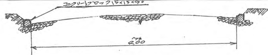
道路断面图 S. 1/40
