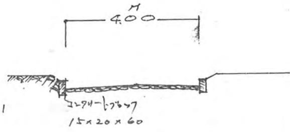
道路断面圖 S=1:100
