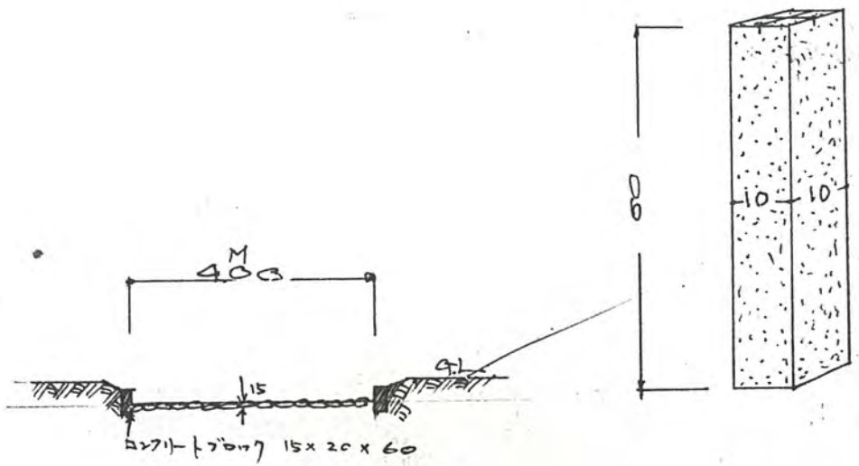
標 杭 图
