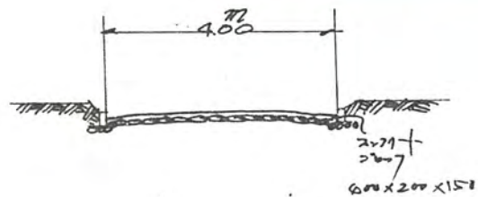
道路断面圖 1/100
