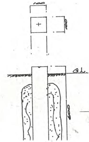
標石断面図 5/10
