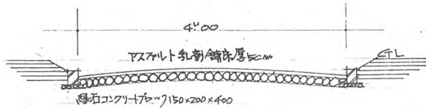
道路断面図 \frac{1}{50}
