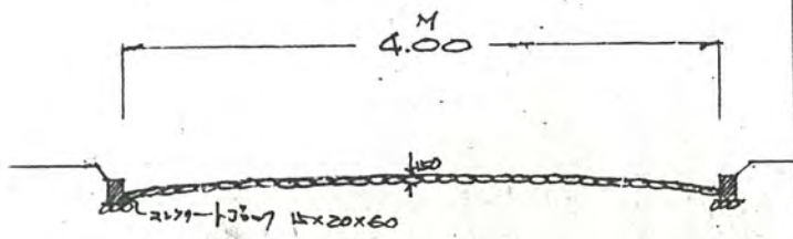
道路断面図
