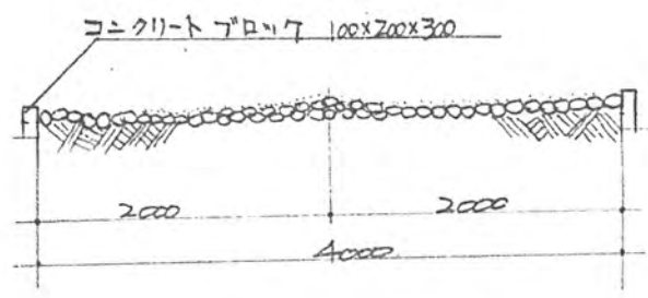
道路断面図 1/50
