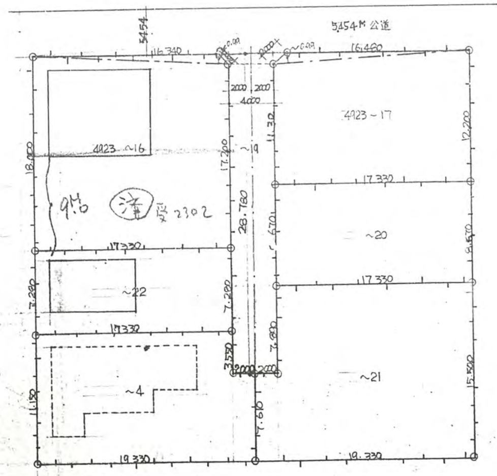
地籍図 5: 1/300
