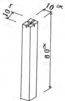
コンクリート製標石
