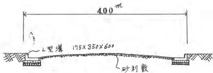
道路断面図
