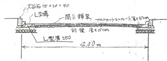
道路断面図 S \sim 1/50
