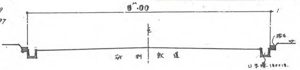
道路境界標石図 S-1:100
